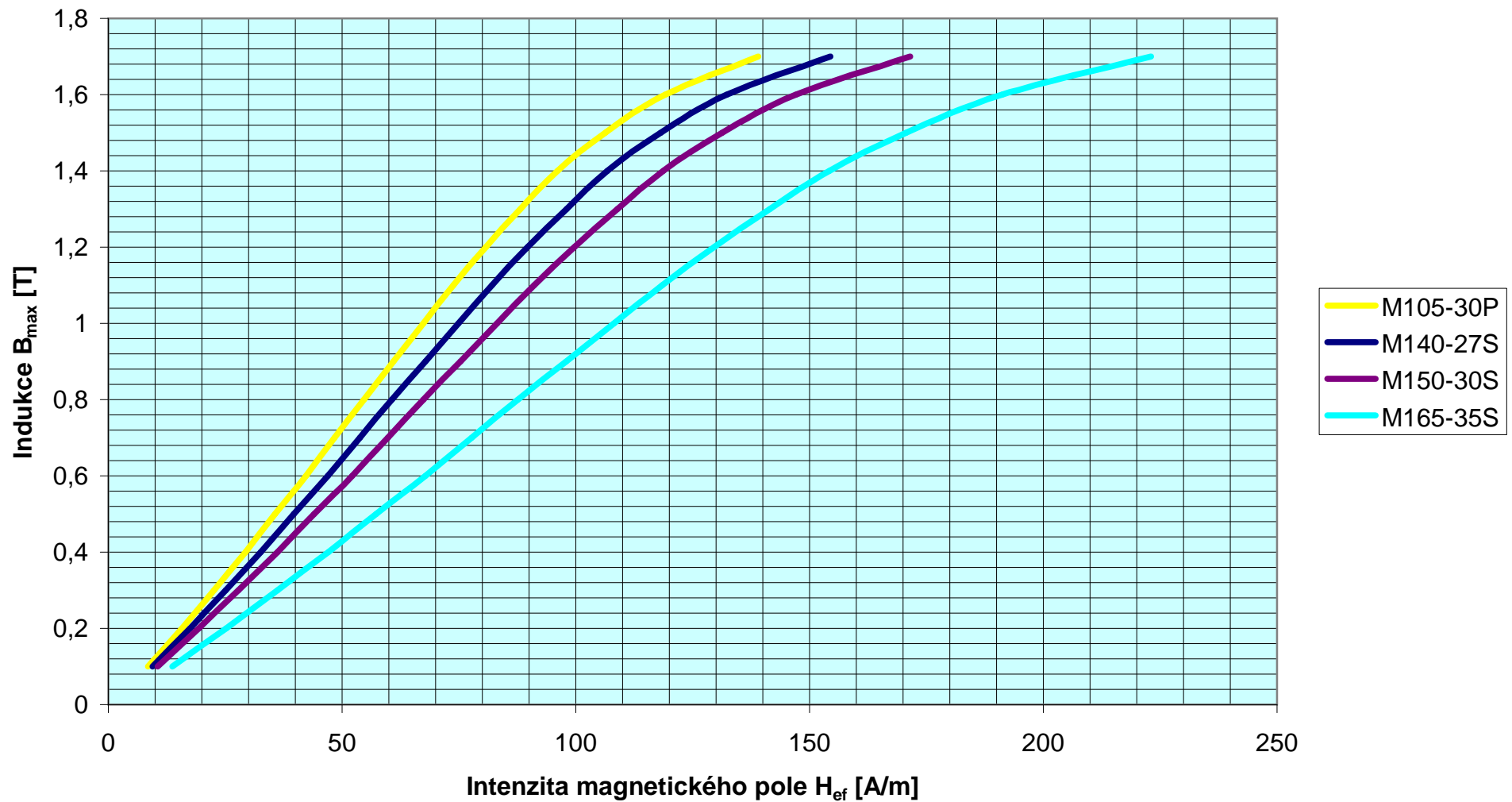
Materiálová charakteristika B_{\max} = f(H_{\text{ef}}) - dělené C-jádro, kvalita "A", 50Hz
